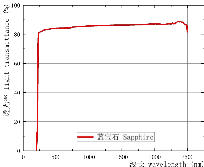
蓝宝石透光率 Sapphire transmittance (标识代号 identification code: TM-SP-A)
