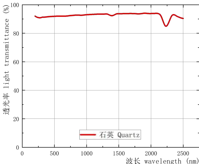
石英透光率 Quartz transmittance (标识代号 identification code: TM-QT-A)
